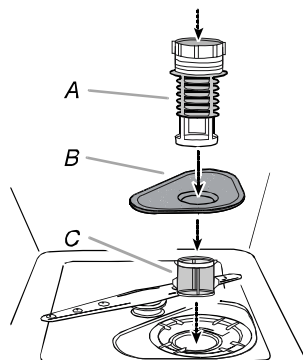
A. Filtre principal B. Crépine métallique C. Filtre fin
